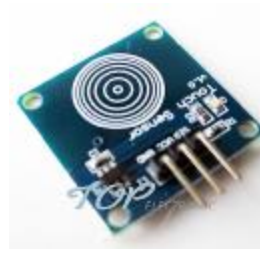
TTP223B Digital Touch Sensor capacitive touch switch module $0.99
